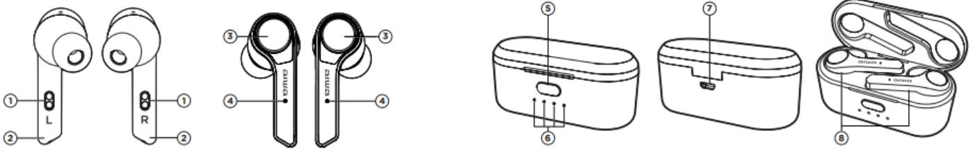
1.Nabíjací kontakty, 2.Mikrofony, 3.Multifunkční tlačidlá, 4.LED indikátory, 5.Test kapacity batérie základne, 6.Indikátor nabíjanie základne, 7.MicroUSB nabíjací port, 8.Pozice pre nabíjanie slúchadiel
