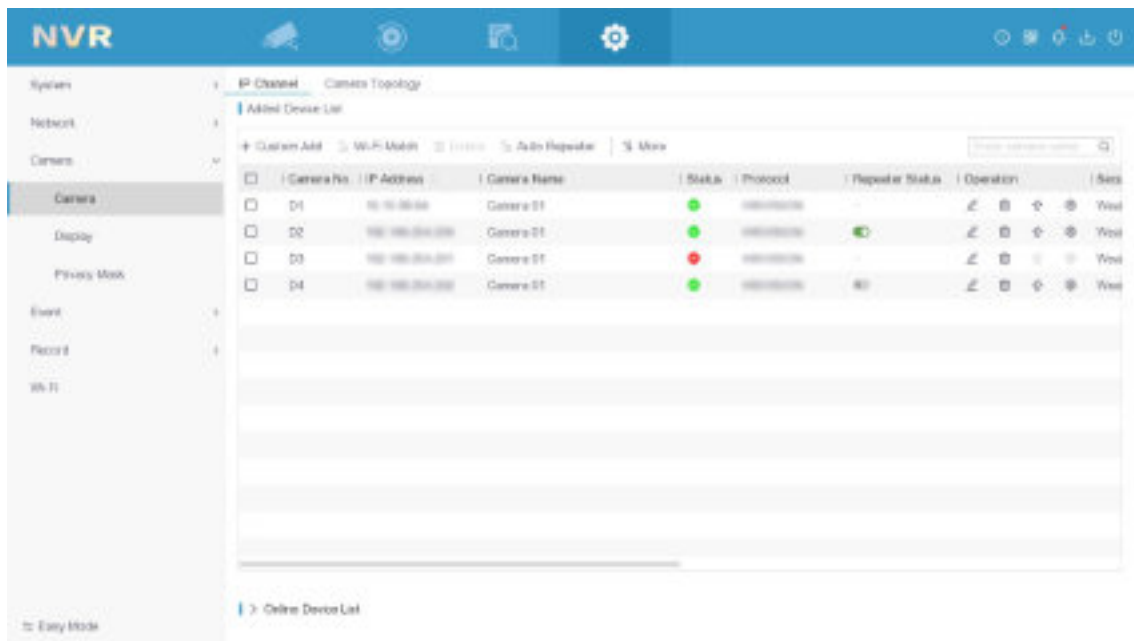
Obrázek 6-8 Konfigurace kamery jako opakovače
