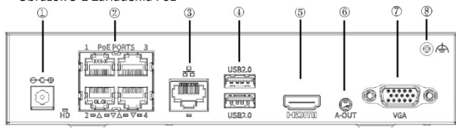
Obrázok 3-2 Zariadenia PoE
