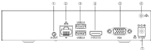
Obrázok 3-1 Zariadenia bez PoE
